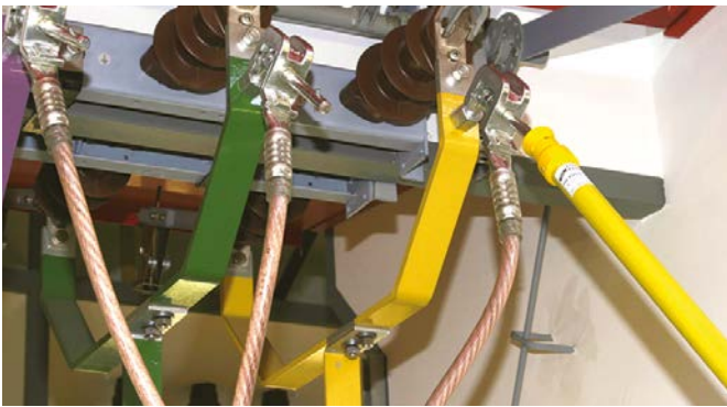
Einbringen einer Erdungs- und KurzschlieÙvorrichtung mit einer Erdungsstange.
