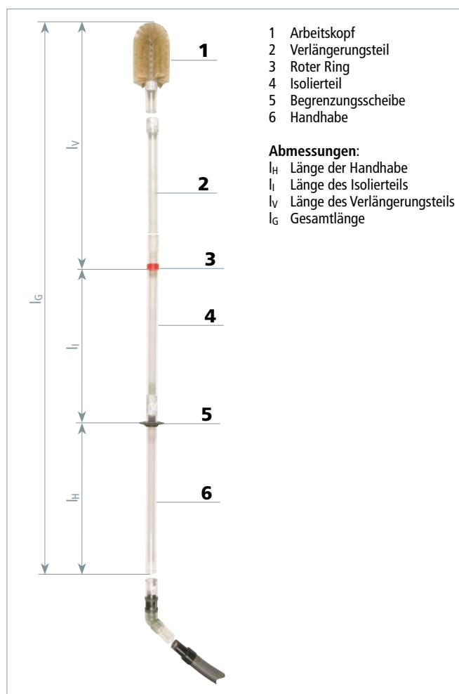
Prinzipdarstellung
