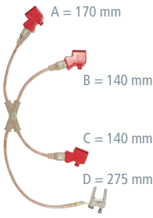
EuK-Vorrichtung VI, Erdungsklemme mit Federvorspannung Klemmbereich bis 24 mm und Befestigung über Drehgriff DGF EKV VI. Für Hausanschlusskasten (HAK).
