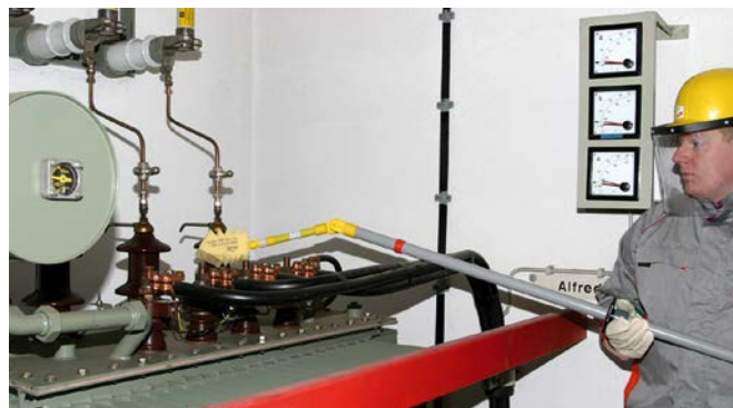
Feuchtreinigung eines Transformators mit dem Feuchtreinigungsset FRS ZK MS.
