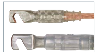
Presskabelschuhe Ausführung PK3: Hakenkabelschuh bis Seilquerschnitt 35 mm 2 auf Anfrage lieferbar.
