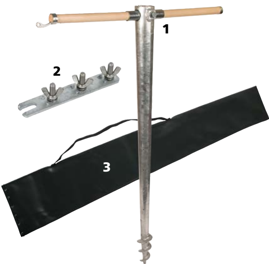
Erdungs-Set Für dreipolige Arbeitserden.
