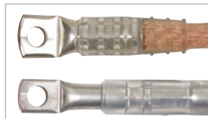
Presskabelschuhe Ausführung PK2: Ohne Ausparung am Kabelschuh für Anschleißteile anderer Hersteller auf Anfrage lieferbar.
