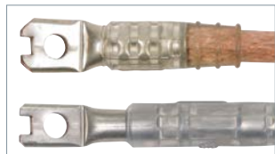
Presskabelschuhe Ausführung PK1: Ausparung am Kabelschuh als Verdrehungsschutz (Standardausführung).
